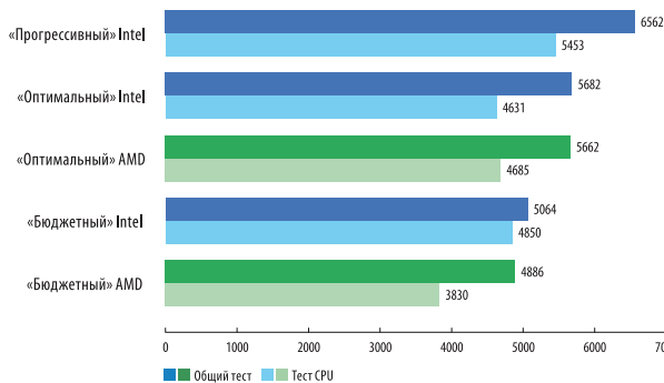
PCMark05, баллы
